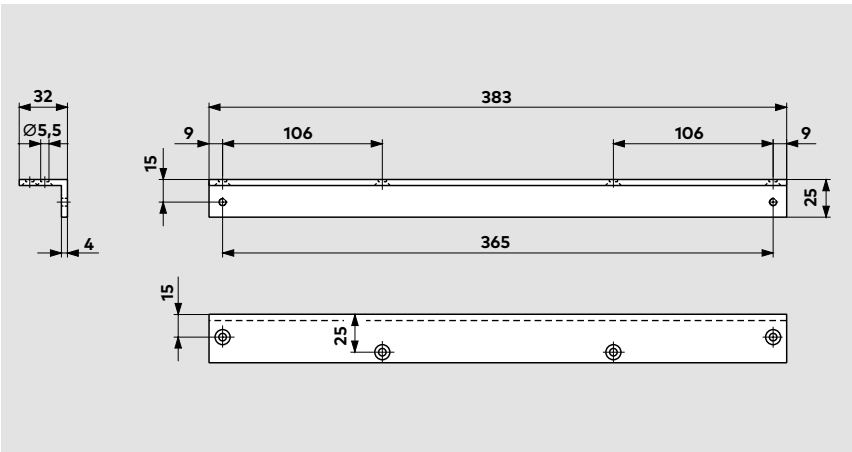
Угловая монтажная пластина для скользящего канала для установки на дверную коробку с четвертью со стороны, противоположной петлям.
