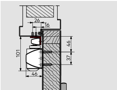
Угловая монтажная пластина для скользящего канала для установки на дверную коробку с четвертью со стороны, противоположной петлям.
