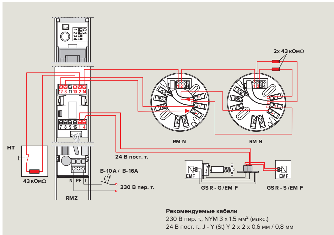
Схема соединений, GSR-EMR XEA с 2x RM-N
