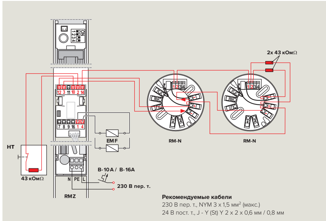
Пример схемы соединений, RMZ XEA с 2x RM-N
