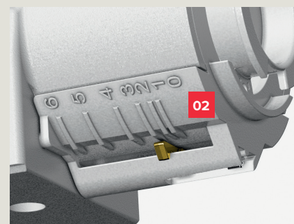
Индикатор в соответствии с информацией о размере в EN 1154 для ширины двери.
