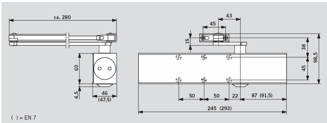
Рис.3. Габаритные размеры доводчика DORMA TS83 Baseline II со складным рычагом.
