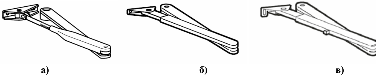
Рис. 2. Варианты складного рычага
